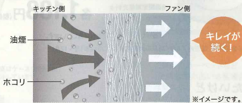
■ダスキンレンジフードフィルター(ガラス繊維タイプ)断面図
